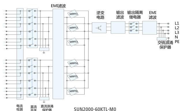
电路框图
