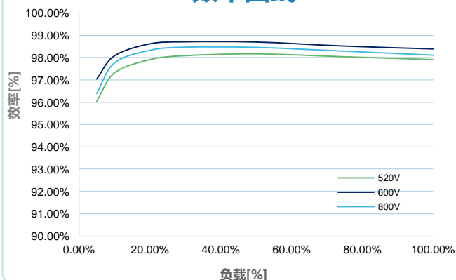
效率曲线
